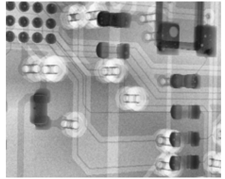
PCB Vias
