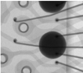
Wire Bonds
